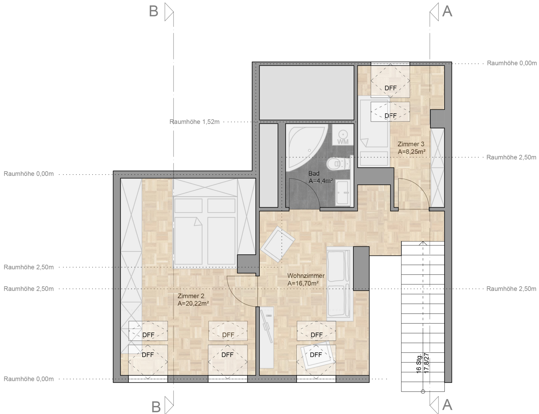
Grundriss: 2.DG
