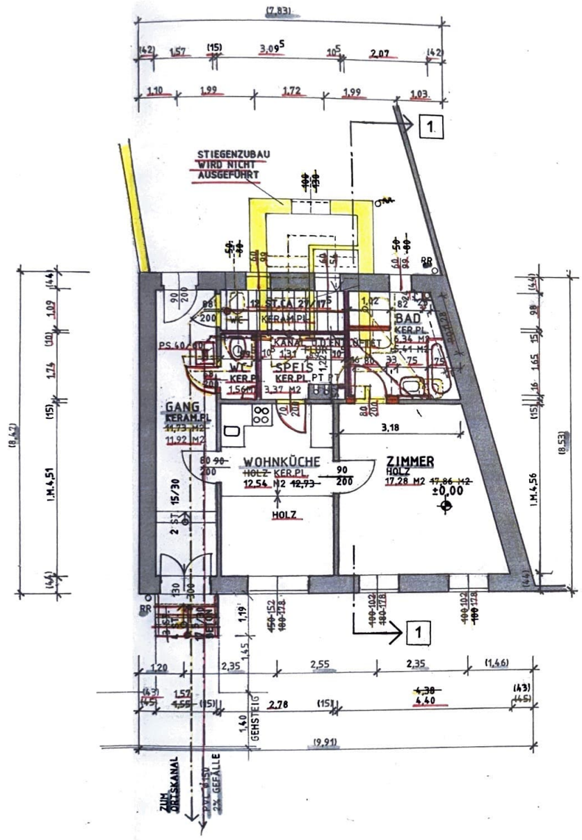
GRUNDRISS ERDGESCHOSS 75 m 2
