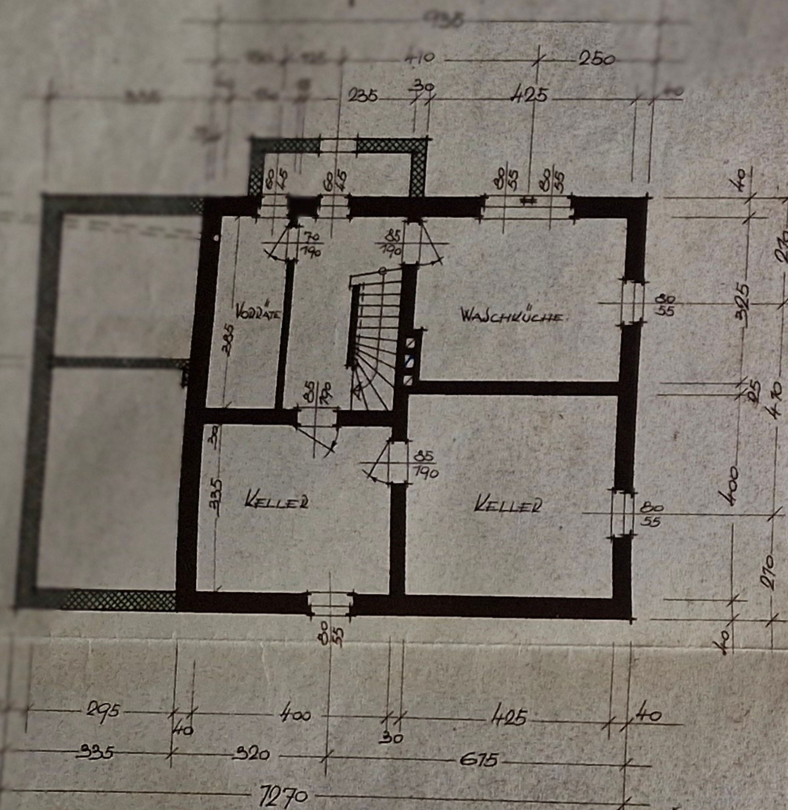
KELLERGRUNDRISS
