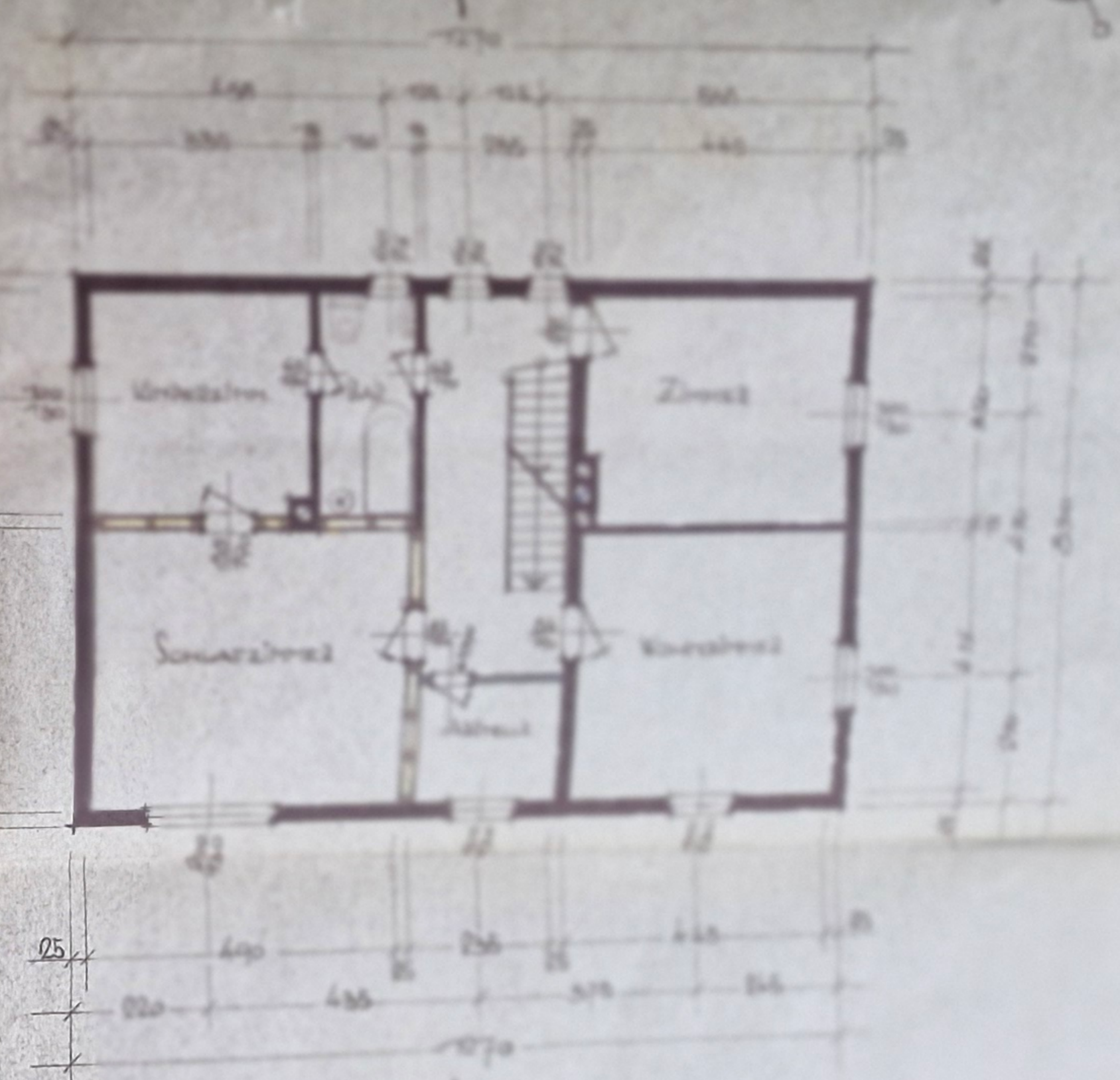
OBERGESCHOSS
