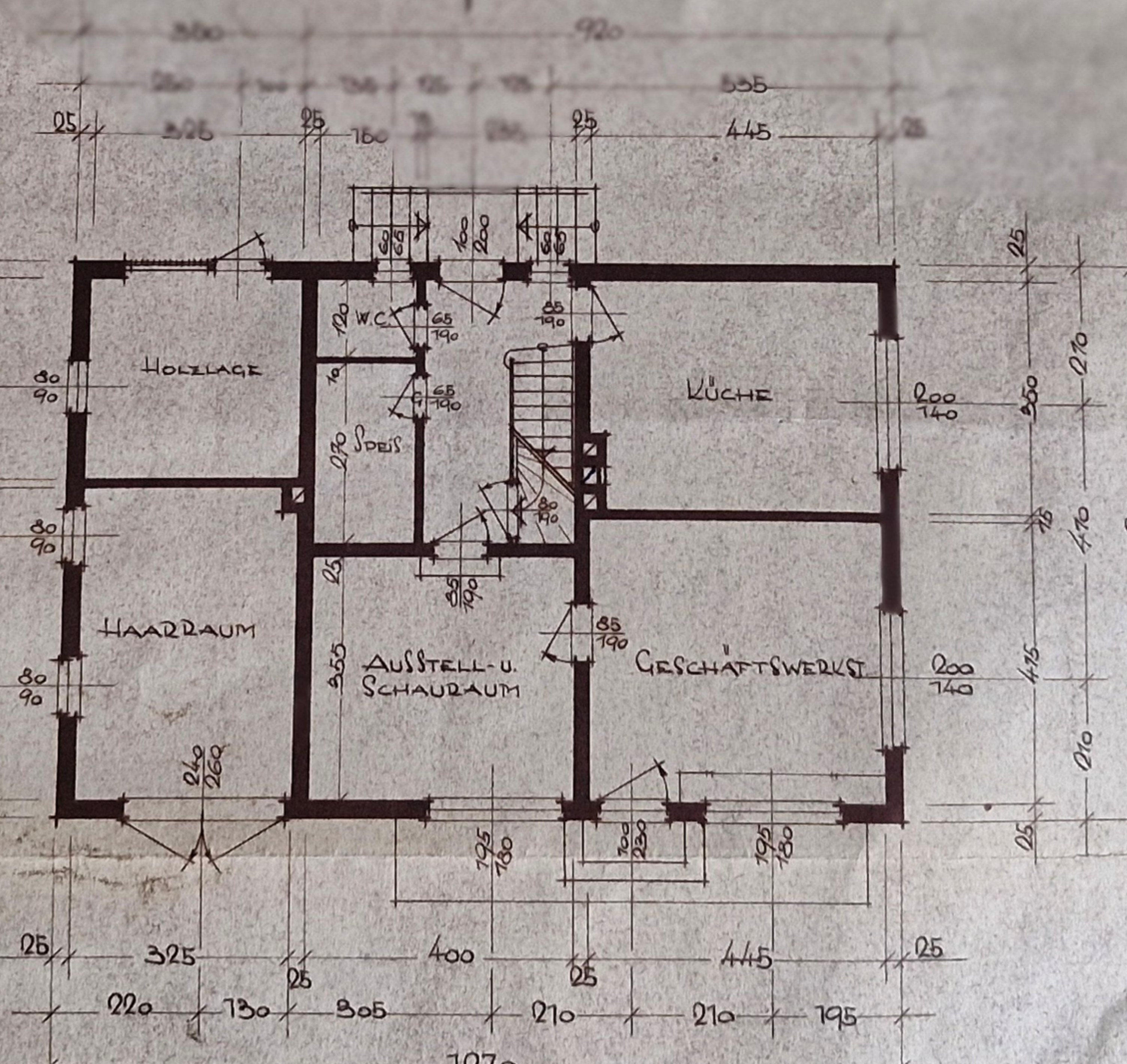
ERDGESCHOSS
