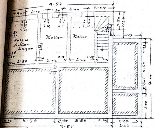
Fundament u. Kellersäume.
