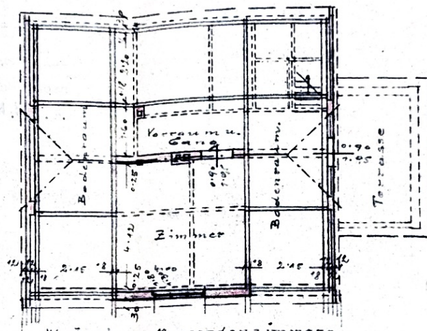
Wehrsatz u. Mansardendach immer Ausbau.
