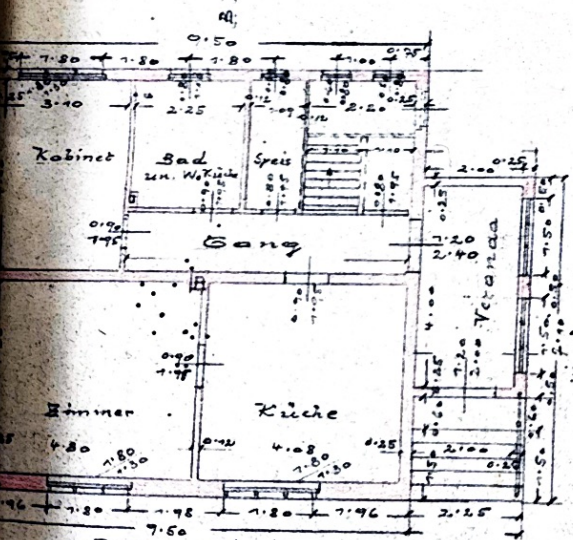
Grundriss.
