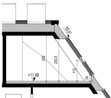
Schnitt 20.B
