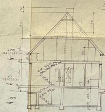
Schnitt A-B
