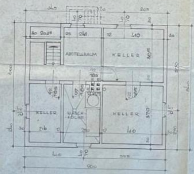
Kellergeschoss
