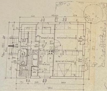
Erdgeschoss
