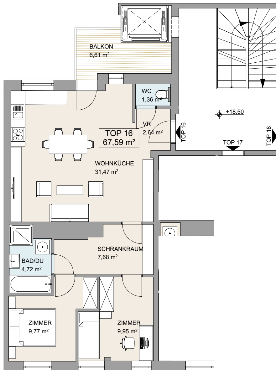
2. DACHGESCHOSS
