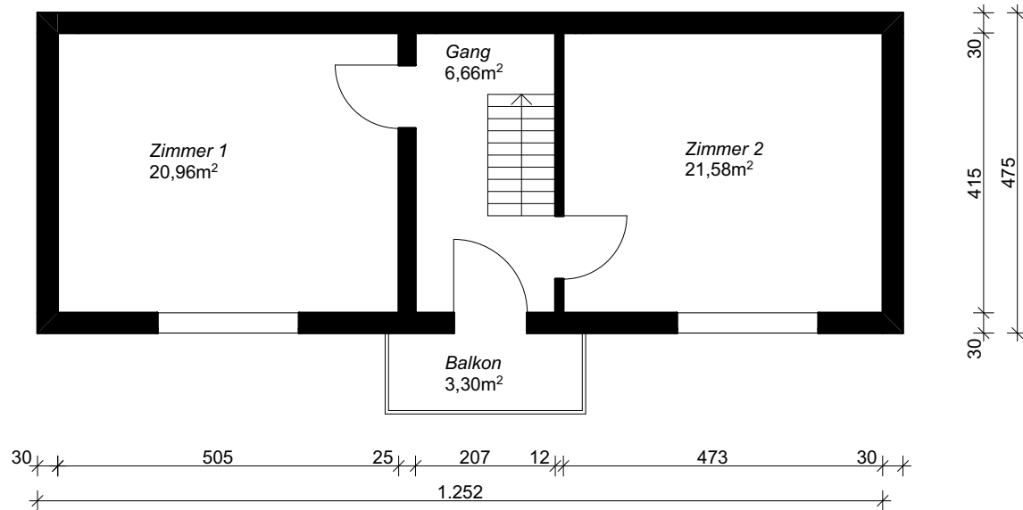
OBERGESCHOSS M 1:100
