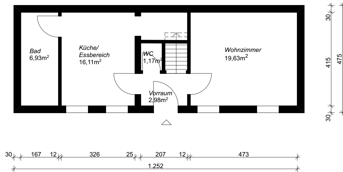
ERDGESCHOSS M 1:100
