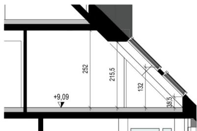
Schnitt 18.A
