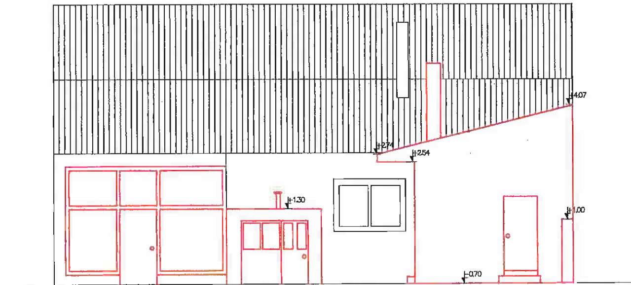
ANSICHT NORDOST
