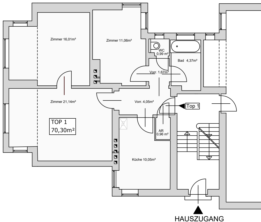
GUNDRISS PARTERRE | MASSSTAB 1:100
