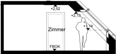
Schnitt
