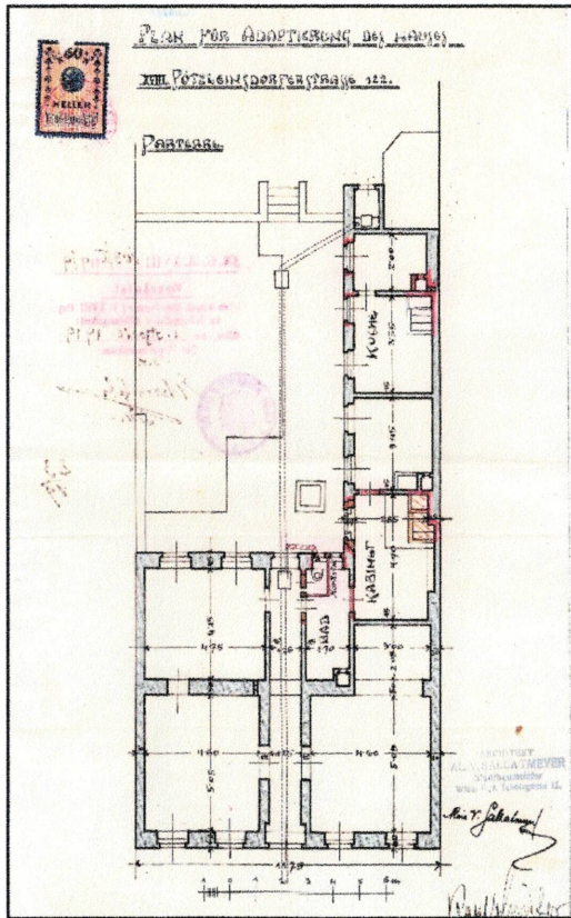
Grundriss Erdgeschoss – Bestandsgebäude
