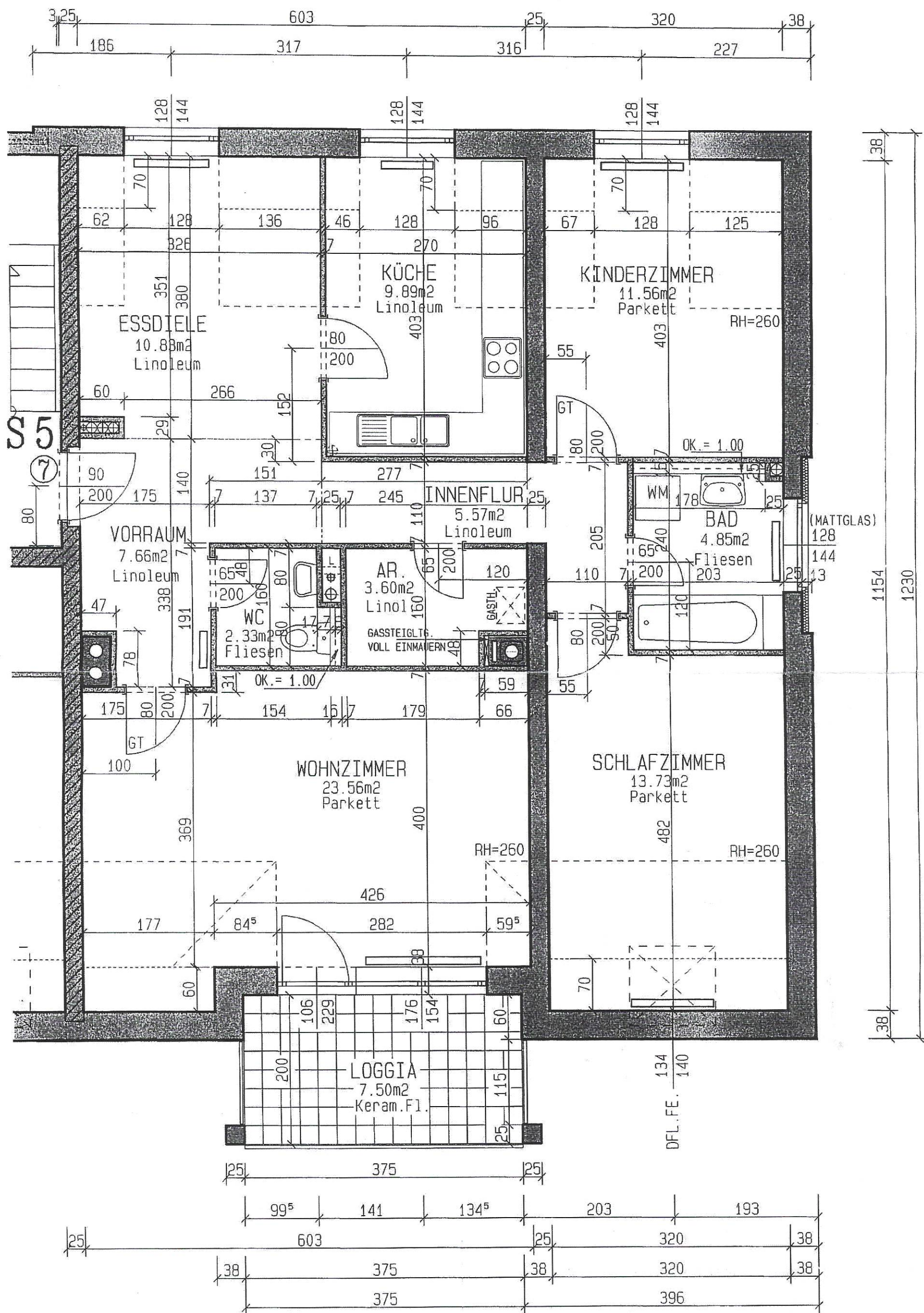
4400 STEYR, HOFERGRABEN 65/7. GRUNDRISS DACHGESCHOSS M - 1:50 STEYR, 24.11.1998
