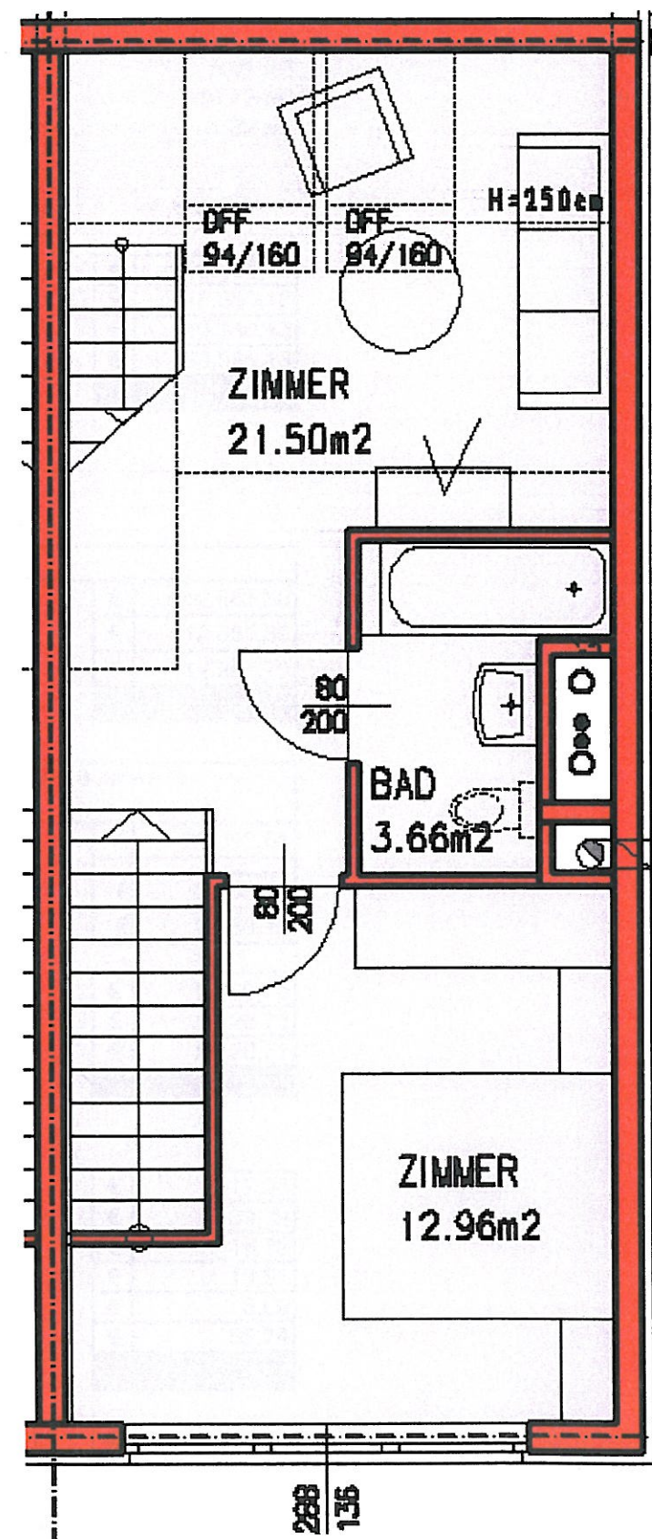
1. DACHGESCHOSS
