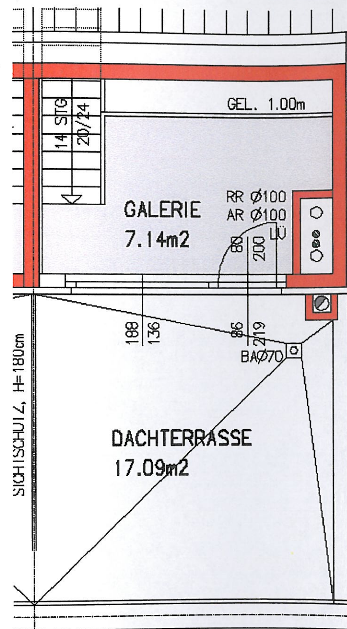
2. DACHGESCHOSS
