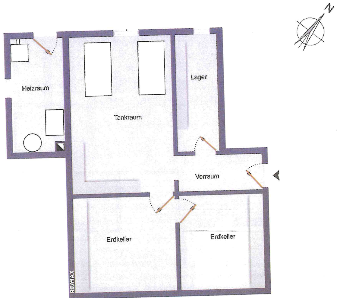
Grundriss Keller
