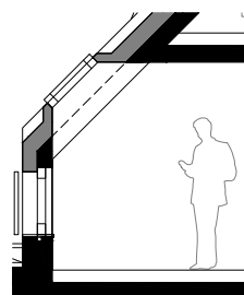
SCHNITT 1-1
