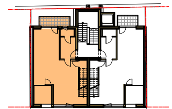
Übersicht 3.OG 1:500
