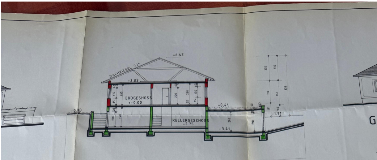
SCHNITT: A-B
