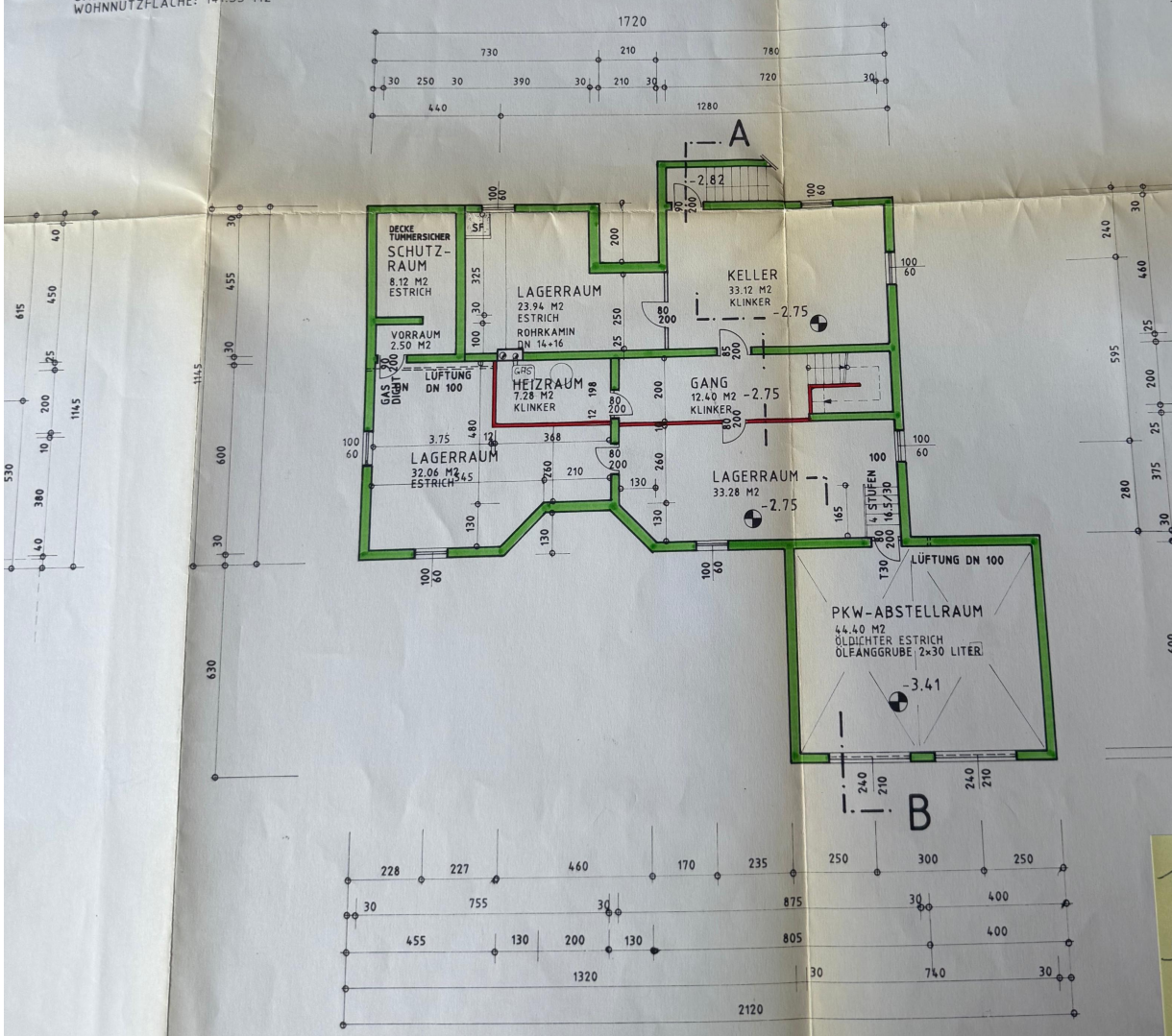
KELLERGESCHOSS
